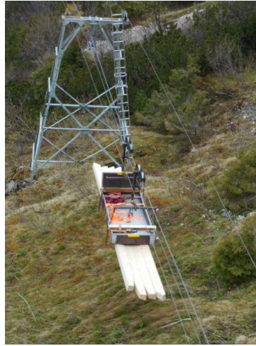
Unsere Materialeilbahn kann auch Überlänge
